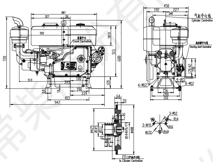
EH24 柴油机外形安装图
