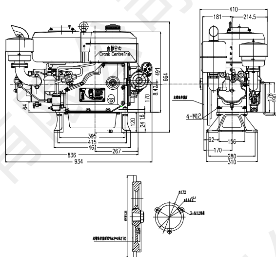
EH20 柴油机外形安装图
