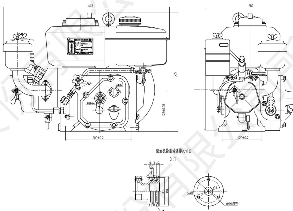
R170B 柴油机外形安装图
