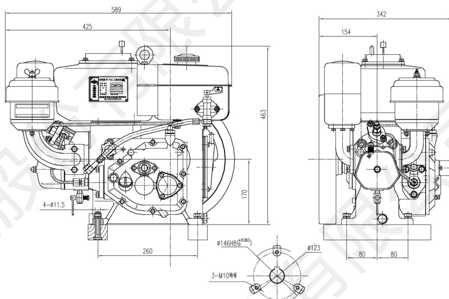
R175B、ZR175 柴油机外形安装图
