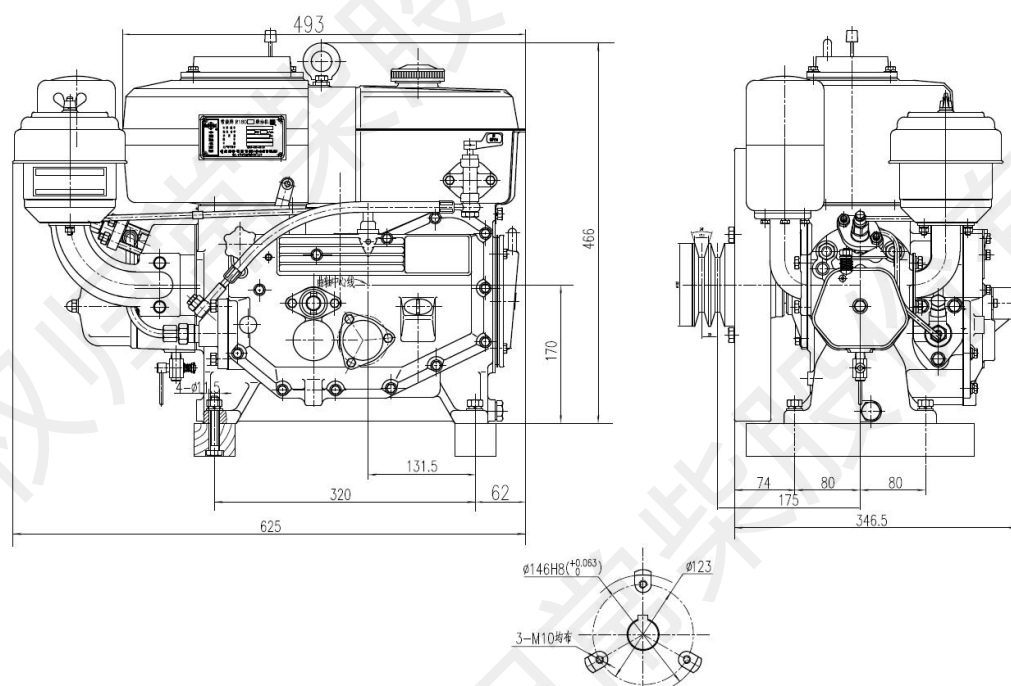
R180、ZR180、Q185 柴油机外形安装图
